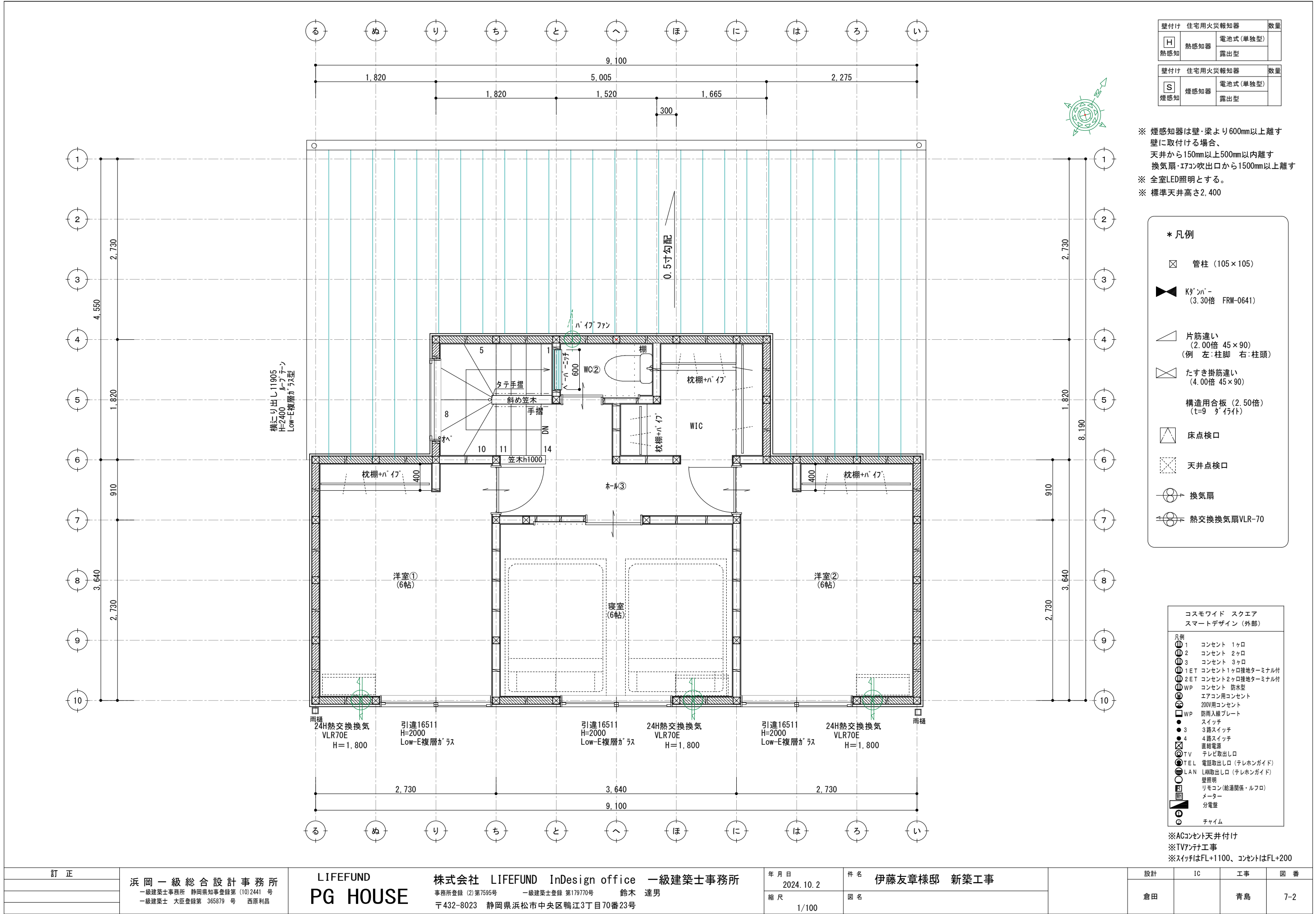
2階電気配線図
